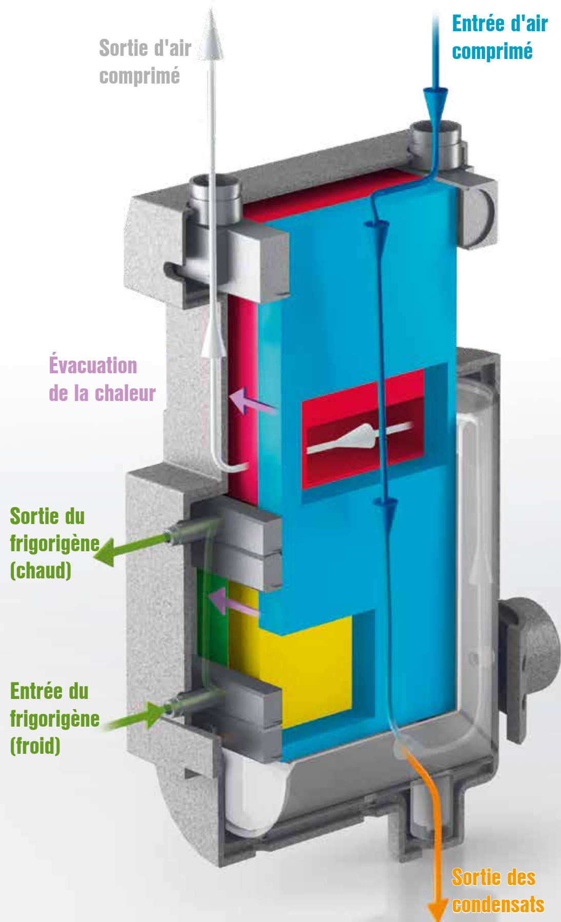
Fig. : SECOPACK LS
